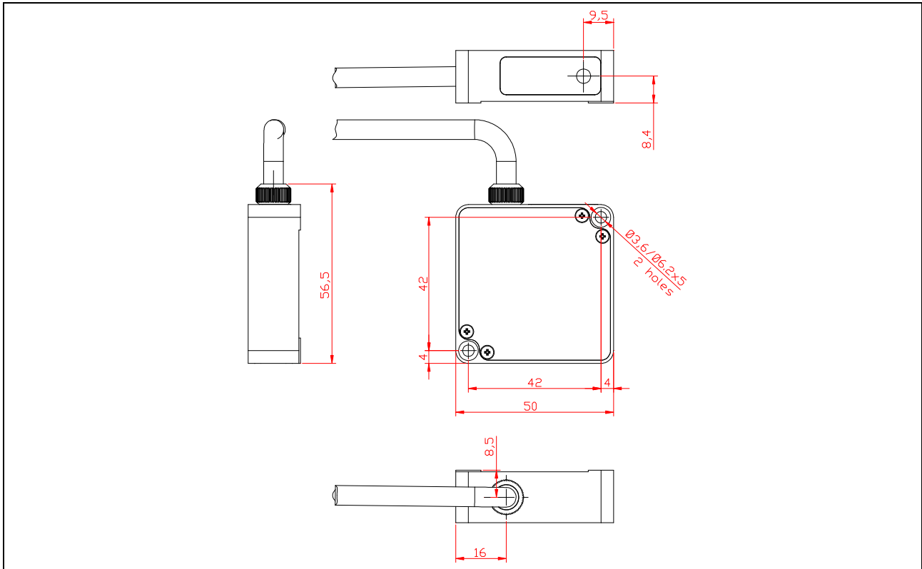
Рисунок 3. Датчик с кабельным вводом
