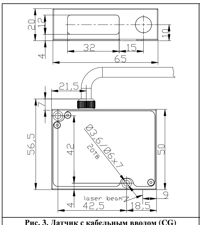
Рис. 3. Датчик с кабельным вводом (CG)
