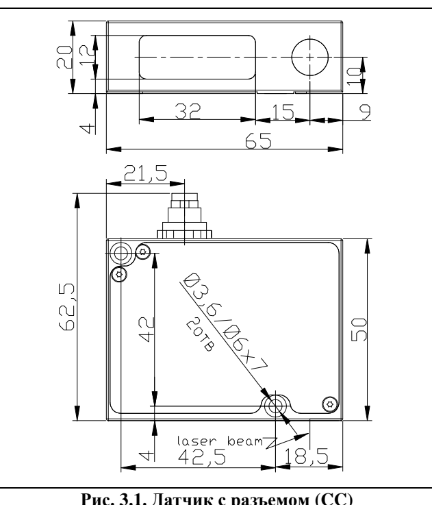
Рис. 3.1. Датчик с разъемом (CC)
